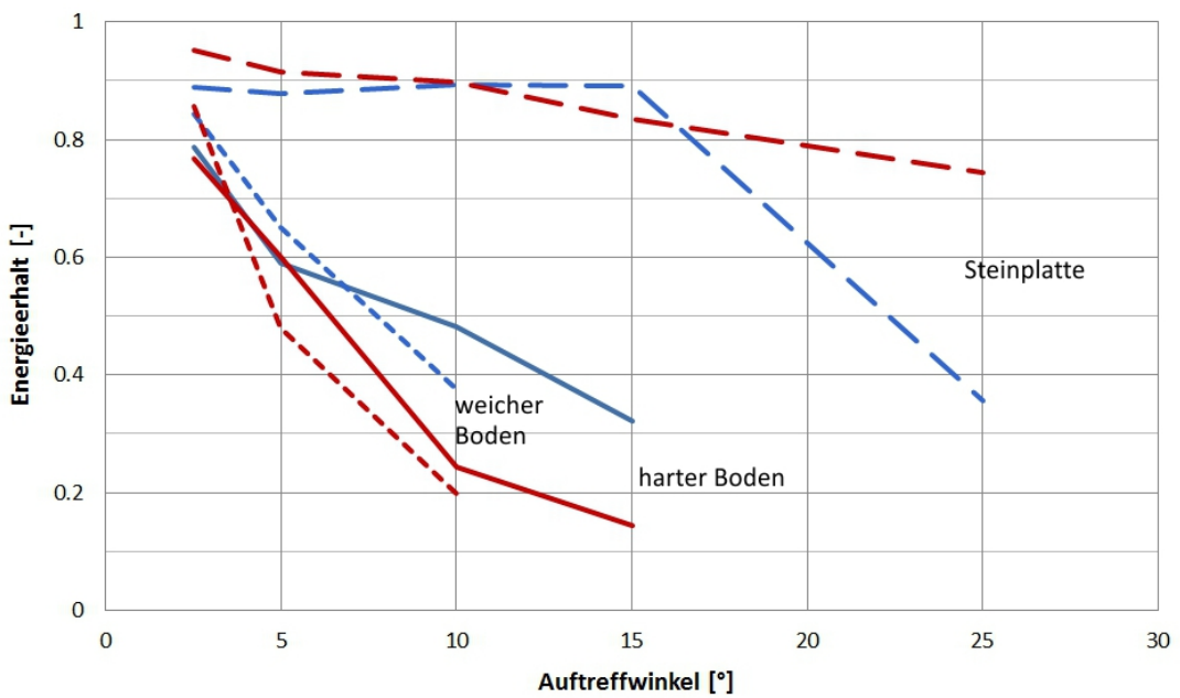
FLG, maximaler Energieerhalt in Abhängigkeit des Auftreffwinkels
