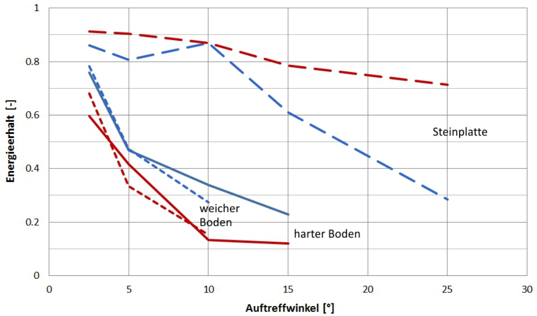
FLG, mittlerer Energieerhalt in Abhängigkeit des Auftreffwinkels
